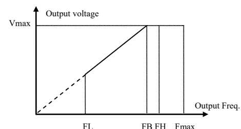
Fig.6-2 F_{max}/F_B/V_{max}0V
