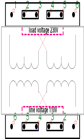
1.5KVA XFMR
