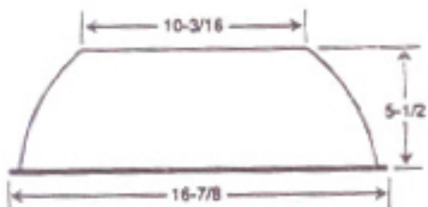
Dome Reflector
