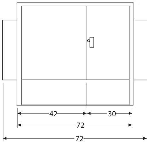
Cabinet/Tank Dimensions
